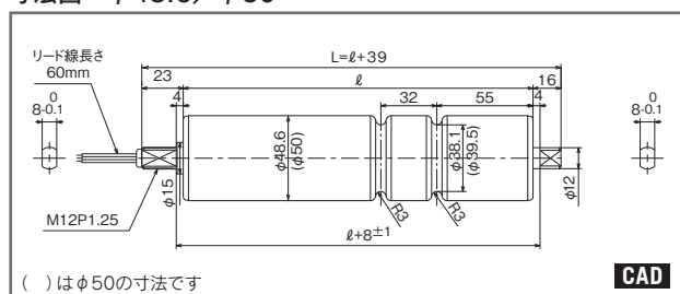
寸法図 φ48.6/φ50
